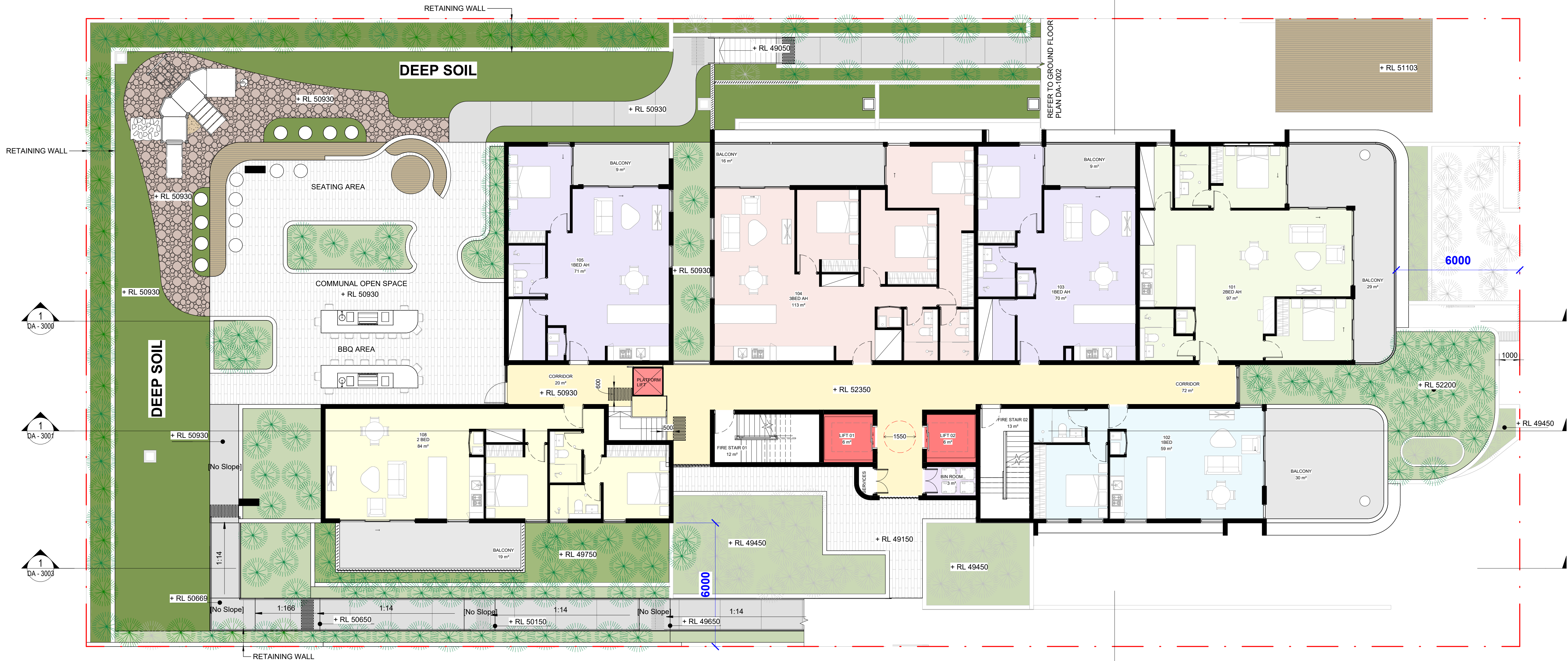
GA LEVEL 01 1 : 100
