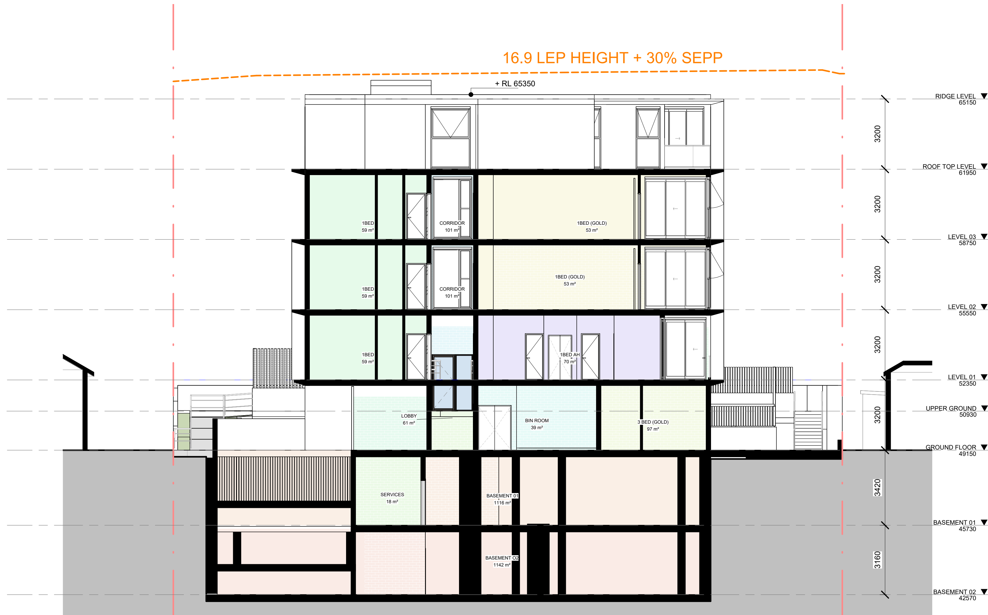
Section 3 1 : 100
